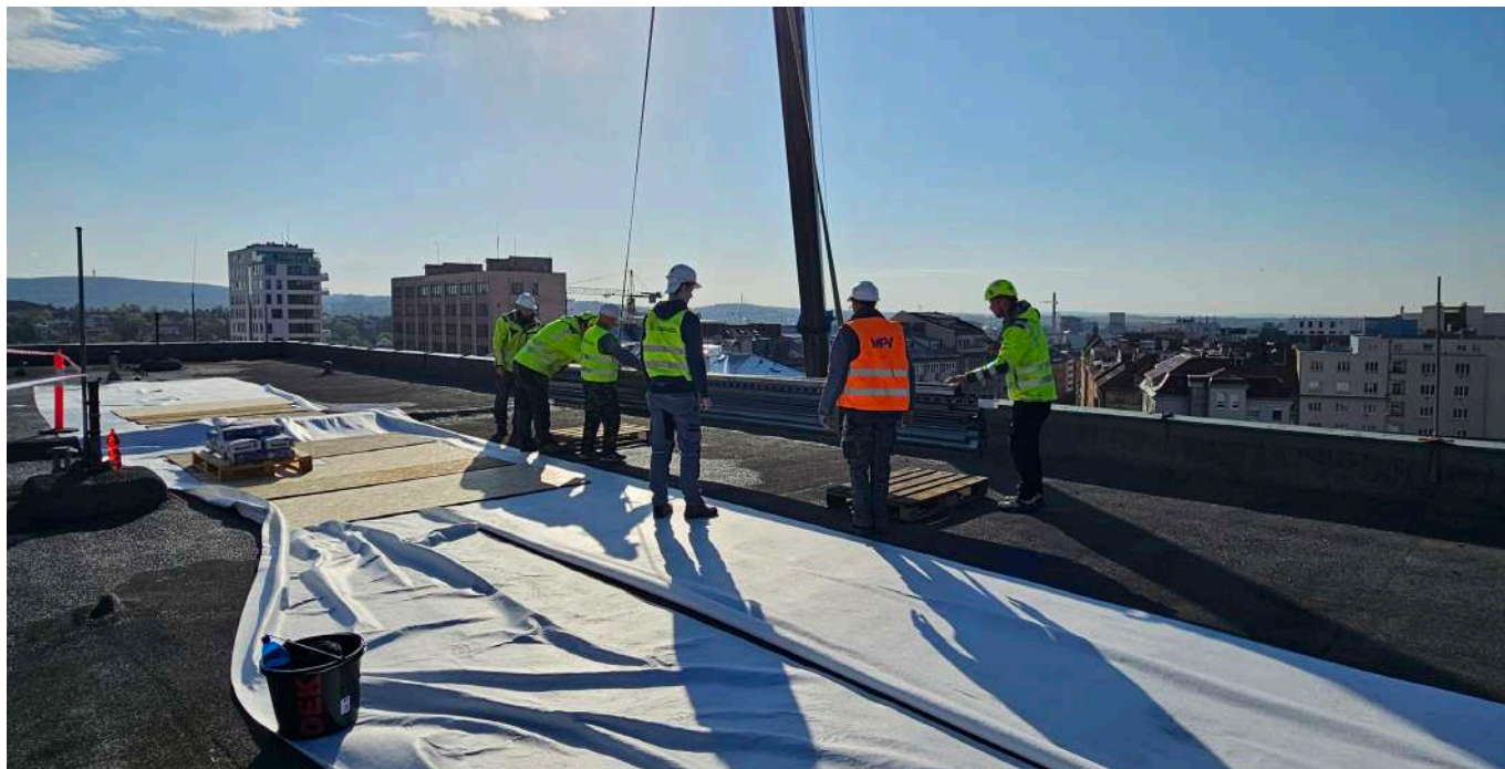
Instalace kondenzačních jednotek na střeše budovy Nejvyššího soudu.
