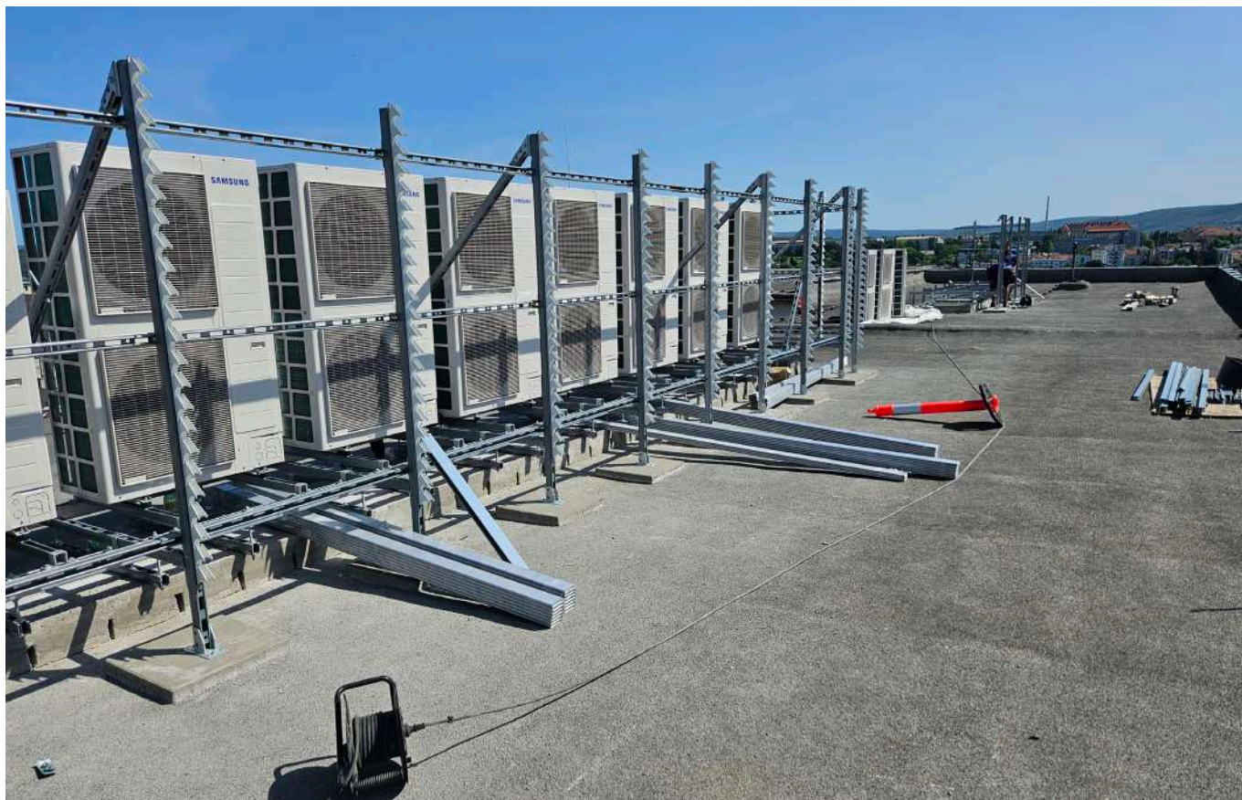
Kondenzační jednotky na střeše budovy Nejvyššího soudu.
